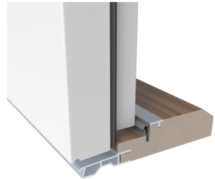
Paksu ovilehti sallii reilun eristevahvuuden. Kalteva kynnyksiprofiili ja ovilehden vesiura ohjaavat kosteuden ulospäin.
